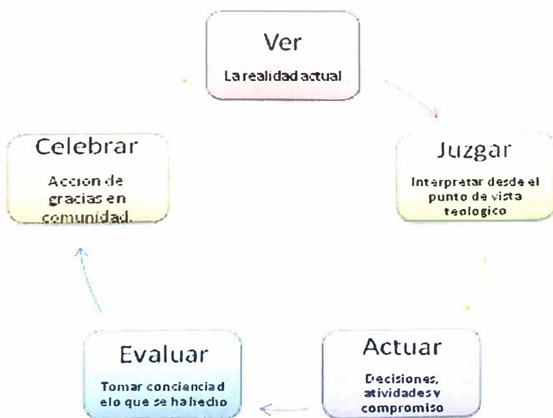
GRÁFICO N°1 MÉTODO INDUCTIVO
