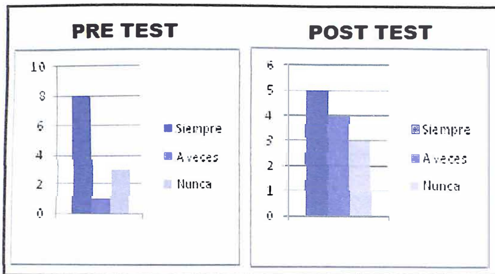
GRÁFICO N° 8 COMPARTIR LIDERAZGO
